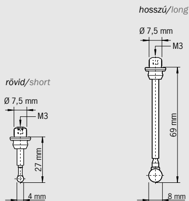
Tapintóbetétek/probe tips
