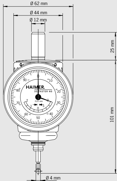
Tapintóbetétek/probe tips
